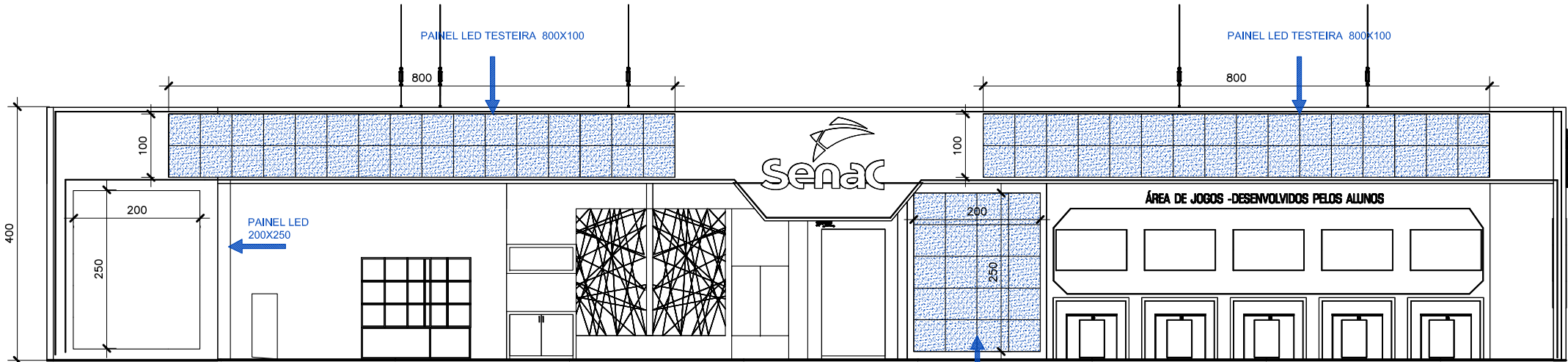
PLANTA ELEVAÇÃO medidas em planta
